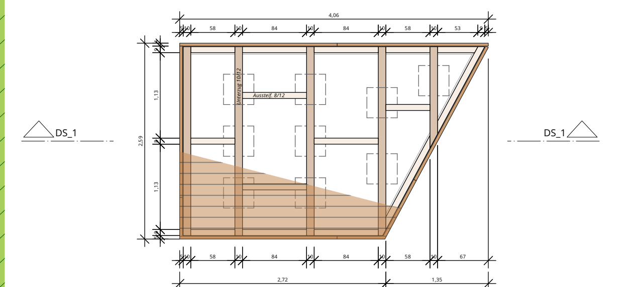
Detail Sitzpodest/Grundriss Unterkonstruktion 1:50
