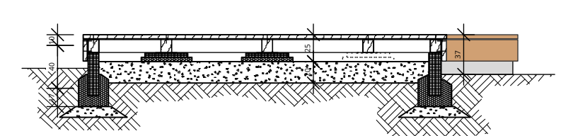
Detail Sitzpodest/Schnitt 1:50
