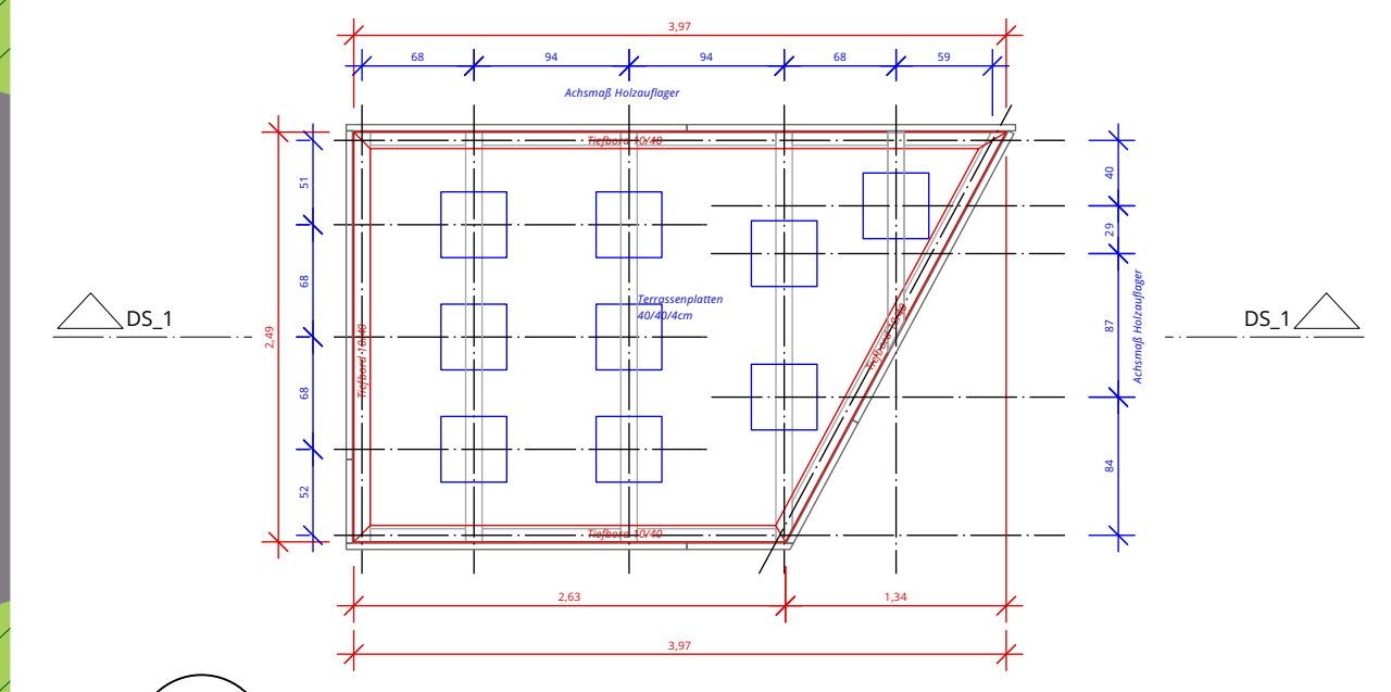
Detail Sitzpodest/Grundriss Auflager 1:50
